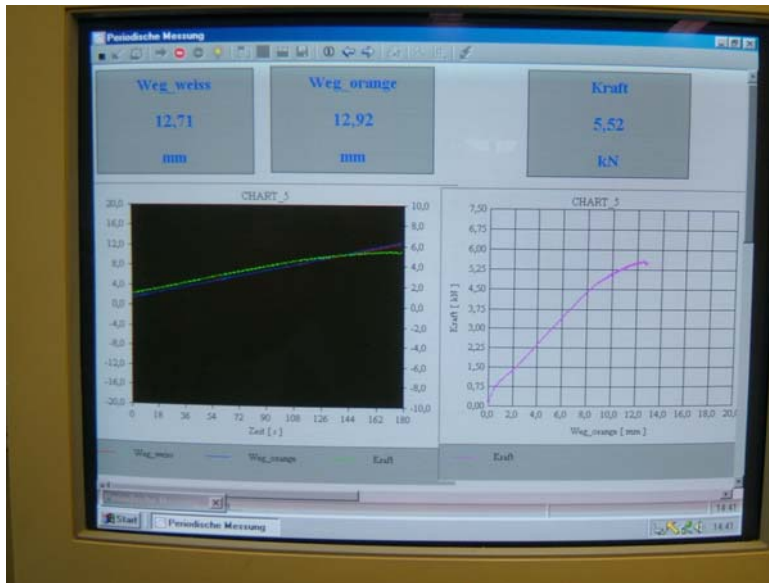
Belastungsdiagramm Beispiel
