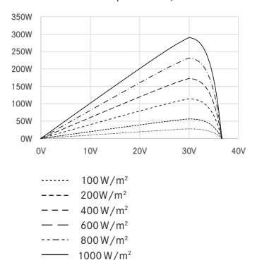
UP-Kennlinie Bsp. LX-290M/156-60+
