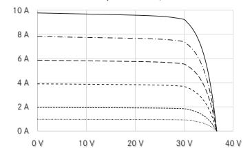
UI-Kennlinie Bsp. LX-290M/156-60+
