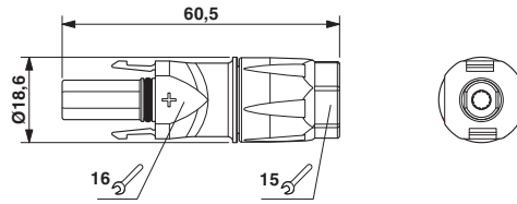
Maßzeichnung
